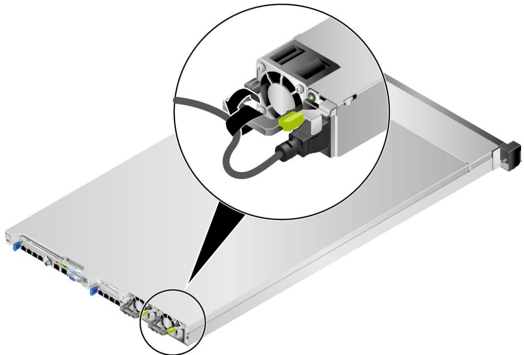
图 6-24 固定电源线缆
