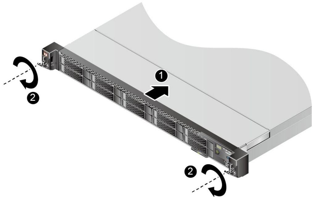
图 6-8 安装服务器
