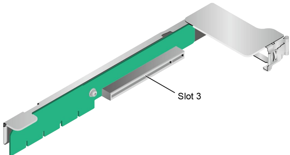
图 3-11 Riser 卡 2 (Slot 3 x16) (板名: BC82PRUW)
