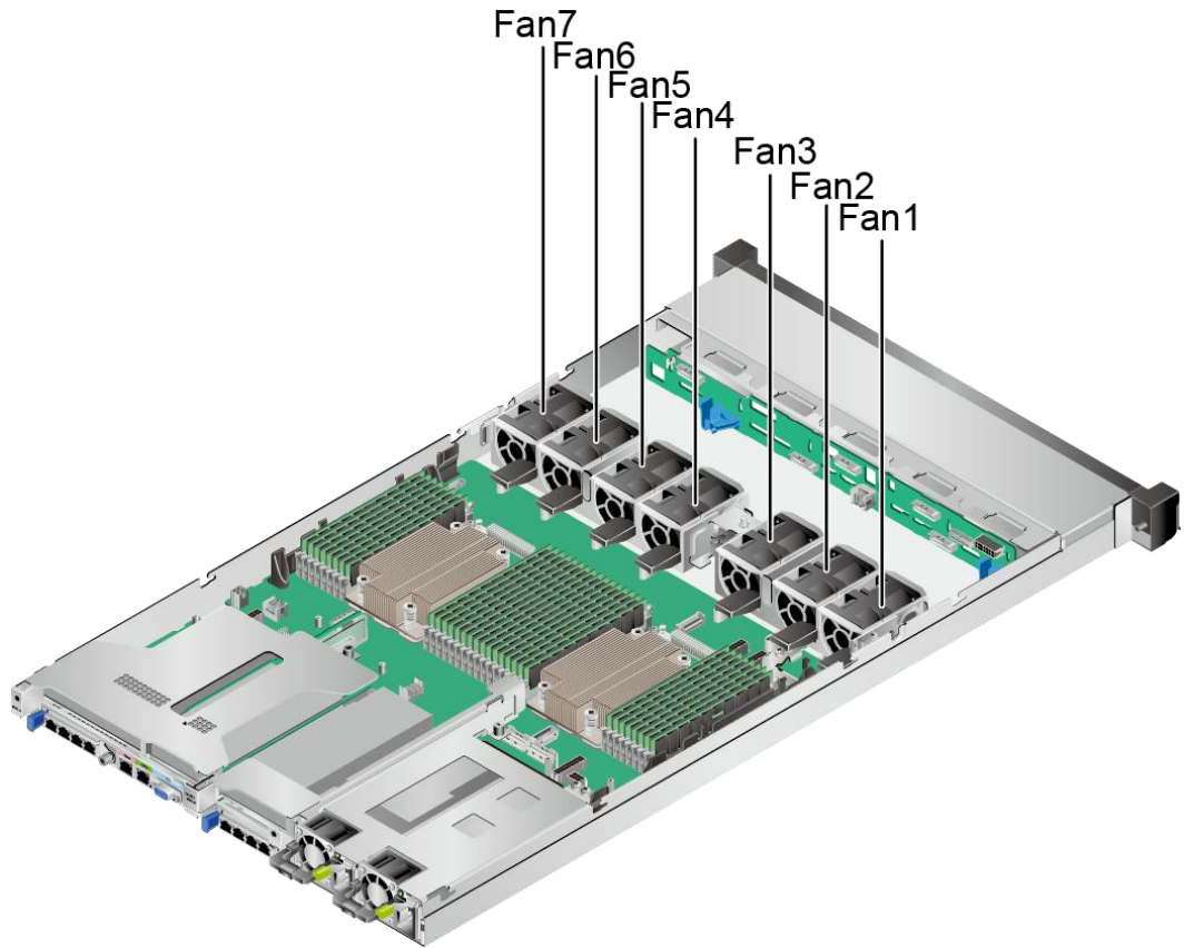
图 3-15 风扇位置图
