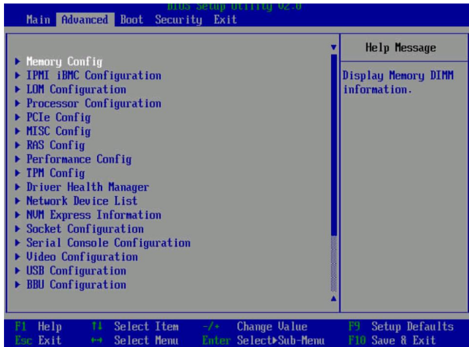
图 6-42 “Advanced”界面
