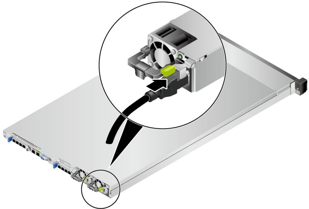
图 6-23 连接电源线缆
