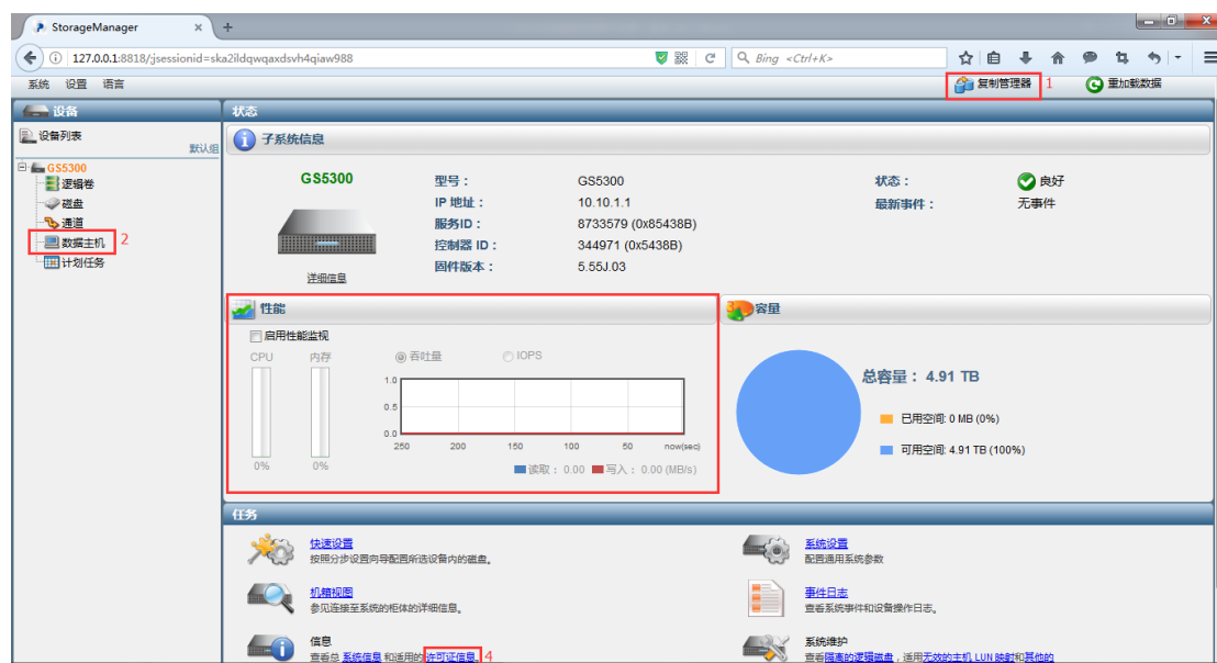
图 3- 91.管理软件高级功能选项
