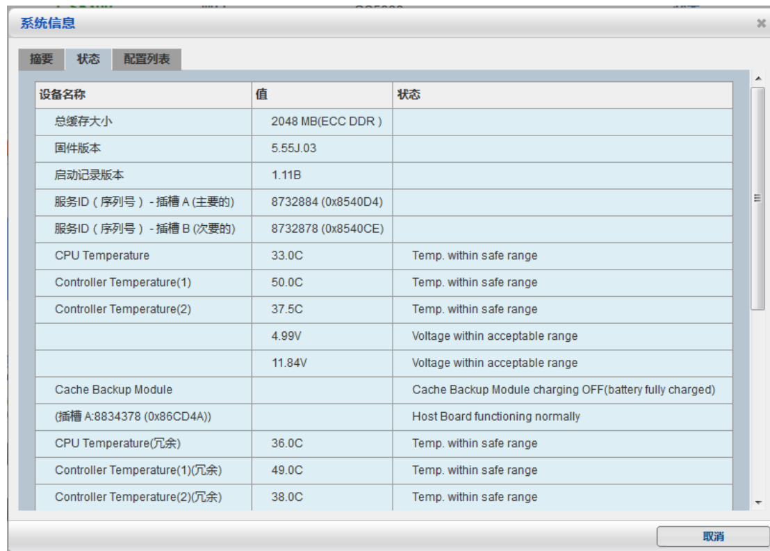
图 3- 39.系统信息-状态
