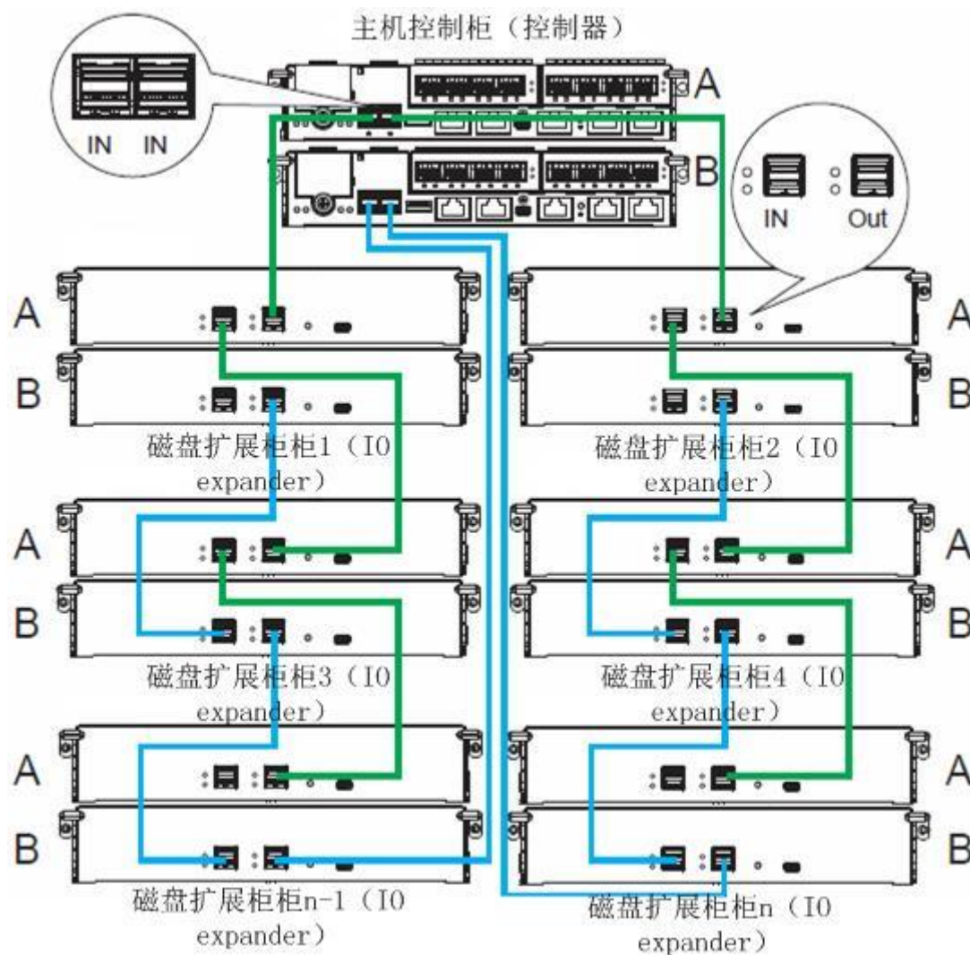
图 1-7.GS6324M 扩展柜连接示意图
