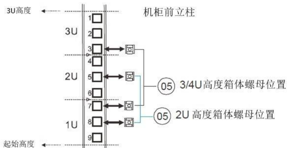
图 2- 2.前立柱螺母安装
