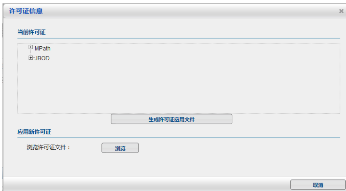
图 3- 96.许可证信息
