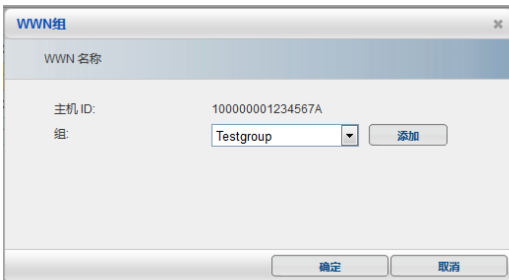
图 3- 63.创建主机组
