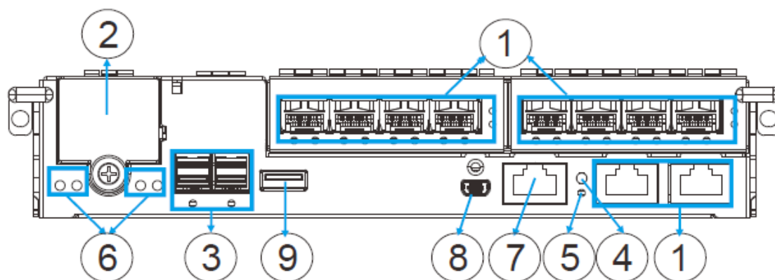
图 1-6.控制器组成
